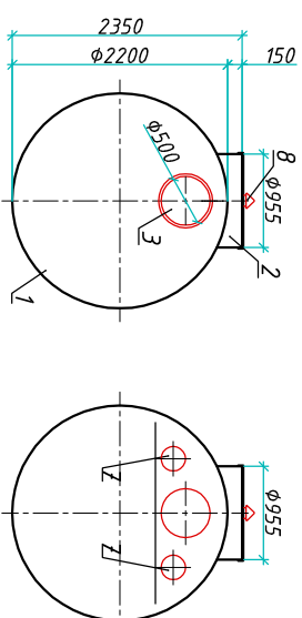
Вид А
